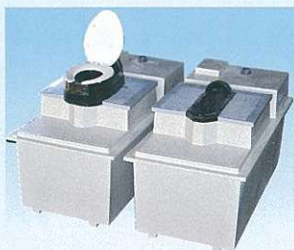
▲便座は洋式と和式の2タイプがあります。 (国交省の定める快適トイレは) 洋式が基準です)
